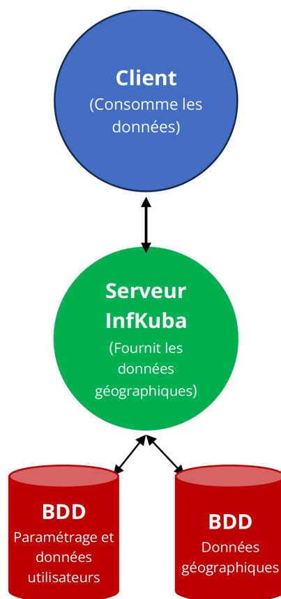
Fig. 5. – Représentation de l’architecture trois tiers d’InfSuite
