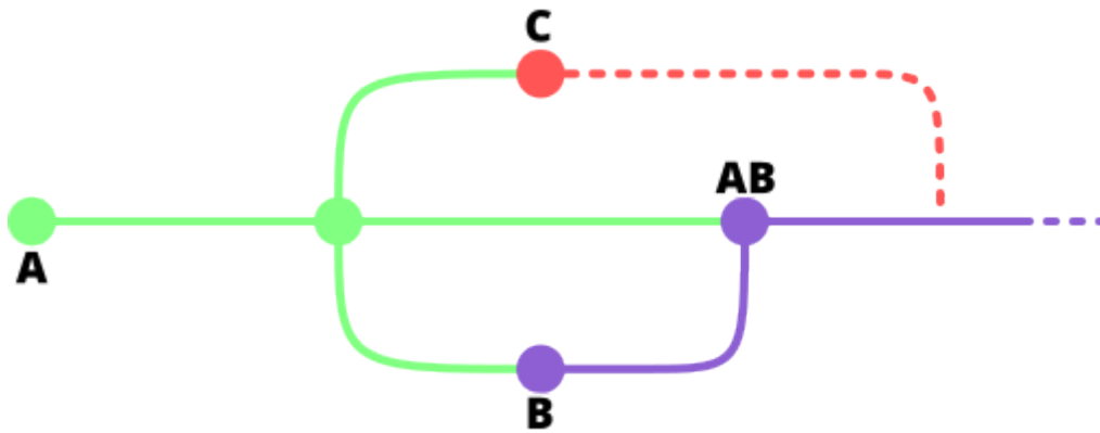
Fig. 6. – Schéma d'un conflit de version entre deux versions d'un document
