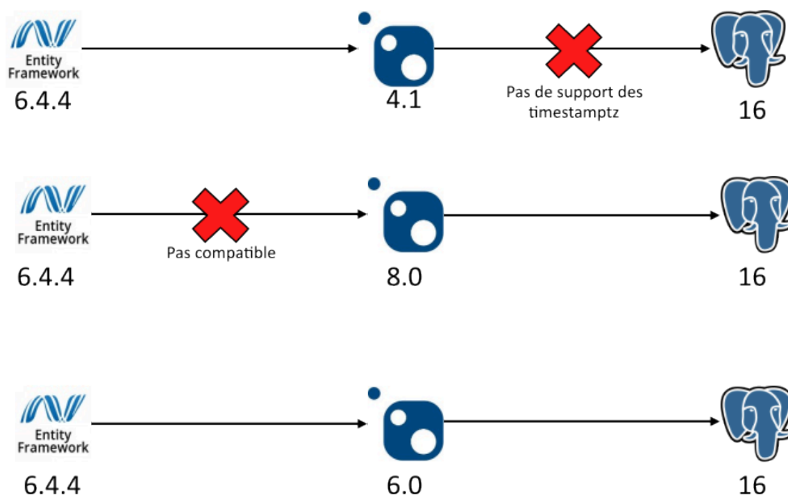
Fig. 8. – Problématique d'incompatibilité entre les différents éléments permettant au serveur et à la BDD d'échanger des informations.
