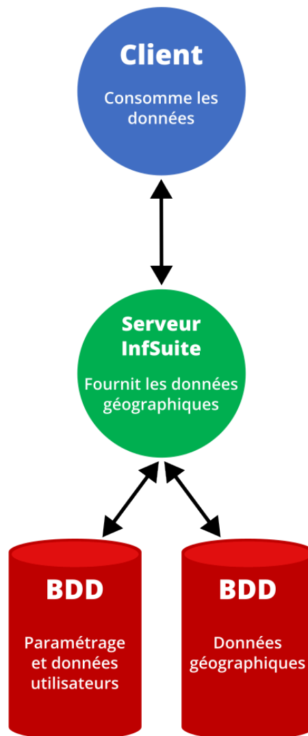
Fig. 5. – Représentation de l'architecture trois tiers d'InfSuite
